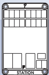
Stationierungstafel Rheinland-Pfalz 90mm x 140mm 4 x 4-teilig, 15mm- Felder, „Station“, ohne Abschnittsfeld
