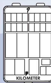
Stationierungstafel Baden-Württemberg 90mm x 140mm 4 x 4-teilig, 15mm- Felder, „Kilometer“
