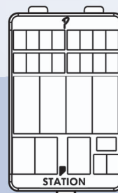
Stationierungstafel Baden-Württemberg 90mm x 140mm 4 x 4-teilig, 15mm- Felder, „Station“
