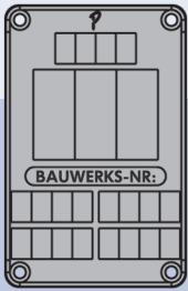
Bauwerkstafel grau 90mm x 140mm x 9mm
