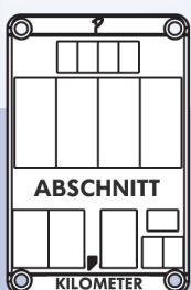
Stationierungstafel Grundplatte 90 mm x 140 mm 1 x 4-teilig, 15 mm Feld „Abschnitt“, „Kilometer“
